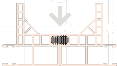
Detalle de unión de guía central
